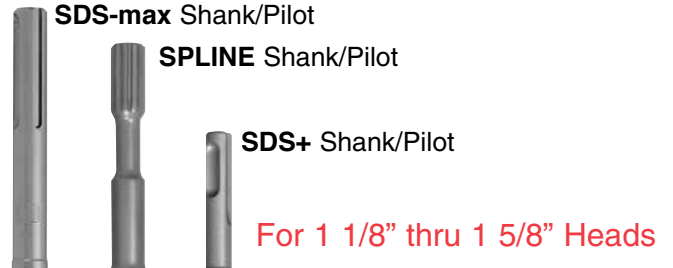
SDS-max Shank/Pilot
